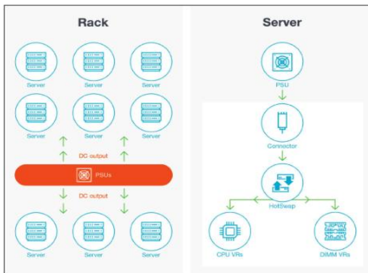
图 9 服务器供电系统示意图
