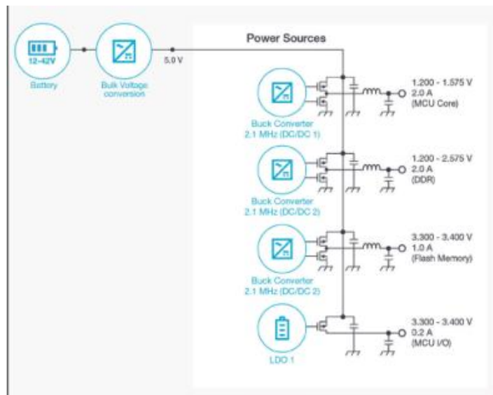
图 8. 汽车信息娱乐供电系统示意图
