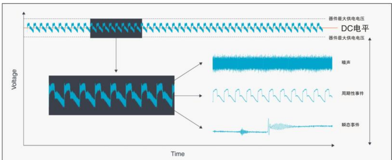
图 1. DC电源噪声的组成成分
