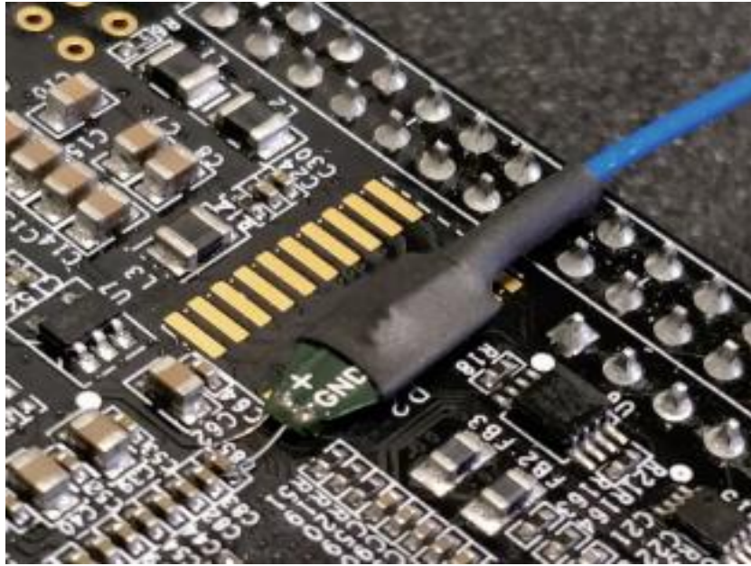
图 4. 透过 0402 解耦电容器连接的 TPR4SIAFLEX 焊接转接头
